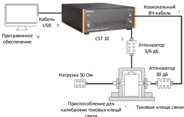
Схема калибровки
