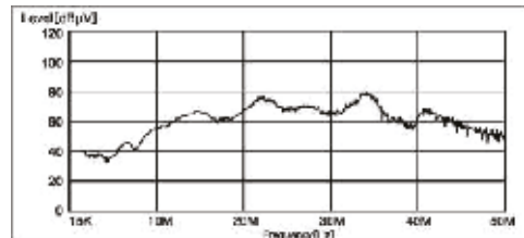
E-ATT = 30 дБ Частотный спектр отрицательного выходного сигнала постоянного тока
