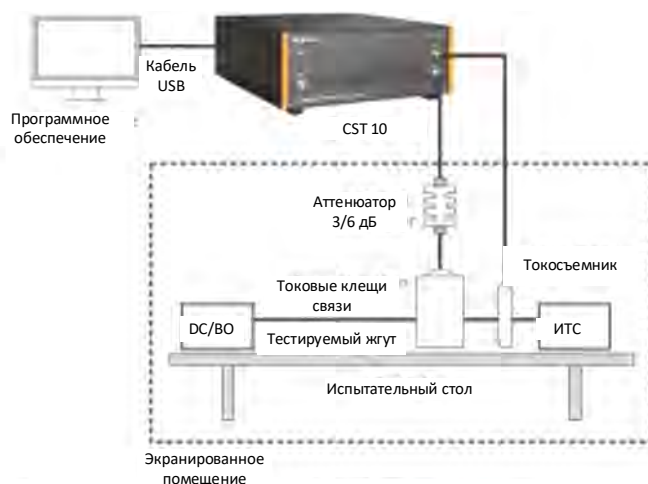
Схема для метода испытаний с обратной связью
