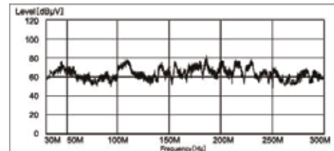
E-ATT = 30 дБ Частотный спектр пространственных помех
