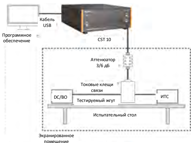
Схема испытаний методом замещения
