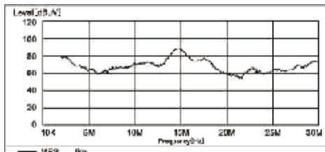
E-ATT = 30 дБ Частотный спектр пространственных помех
