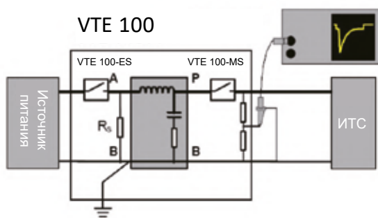
Схема VTE 100
