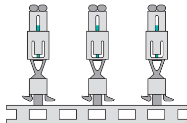
Рис. 10. Расстояние (шаг) между терминалами на несущей полосе
